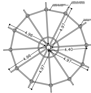
PLANTA SUP. ESQUEMA TERÇAS ESC 1:75
