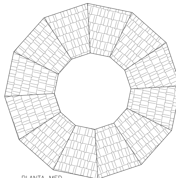
PLANTA MED. COBERTURA ESC 1:75
