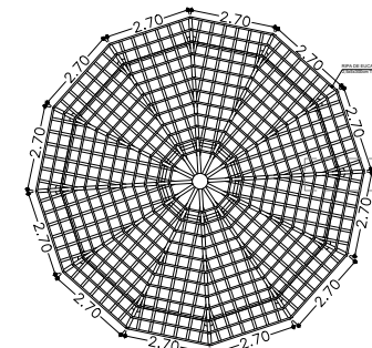
PLANTA SUP. ESQUEMA RIPAMENTO ESC 1:75
