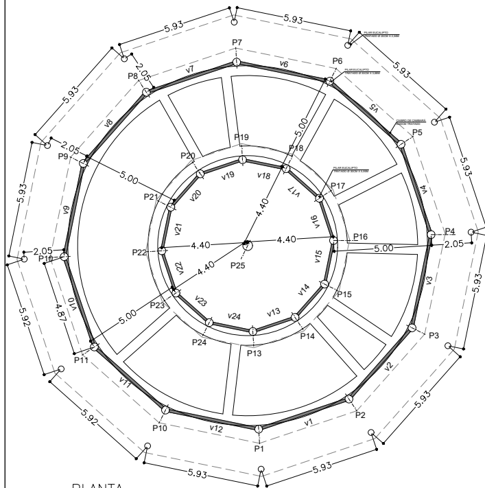
PLANTA PLANTA ESTRUTURAL ESC 1:75
