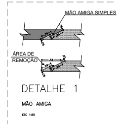
DETALHE FIXAÇÃO MÃO AMIGA ESC 1:50
