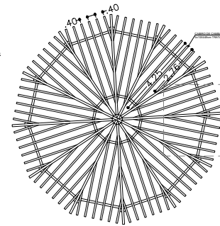
PLANTA SUP. ESQUEMA CAIBROS ESC 1:75
