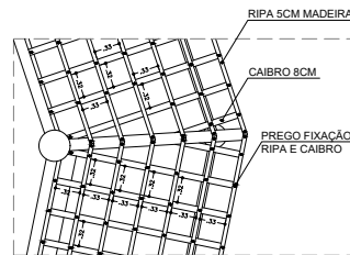
DETALHE 2 FIXAÇÃO RIPAMENTO ESC 1:50
