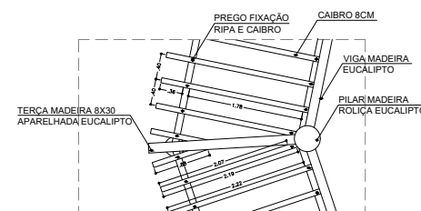
DETALHE 3 CAIBROS ESC 1:50
