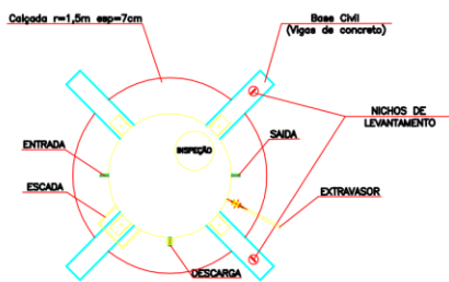
PLANTA BAIXA - GERAL Escala 1:50
